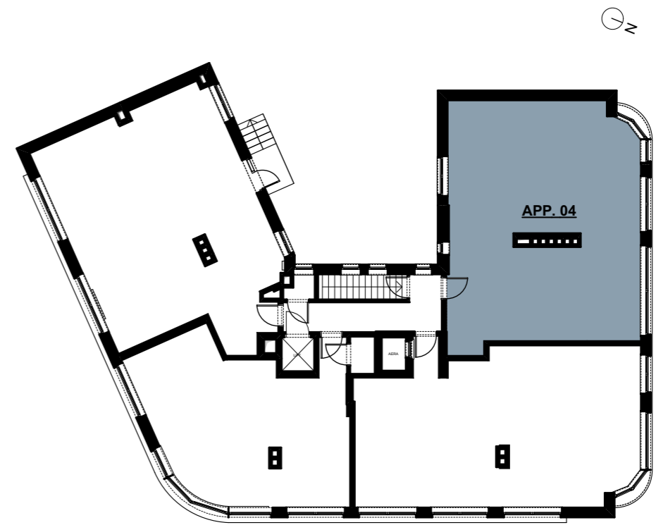
ALGEMEEN PLAN: 4° VERDIEPING
